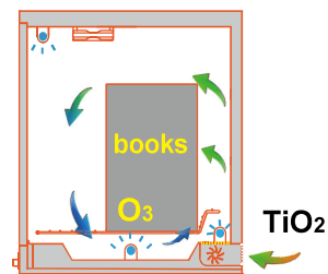
臭氧・光觸媒流向
